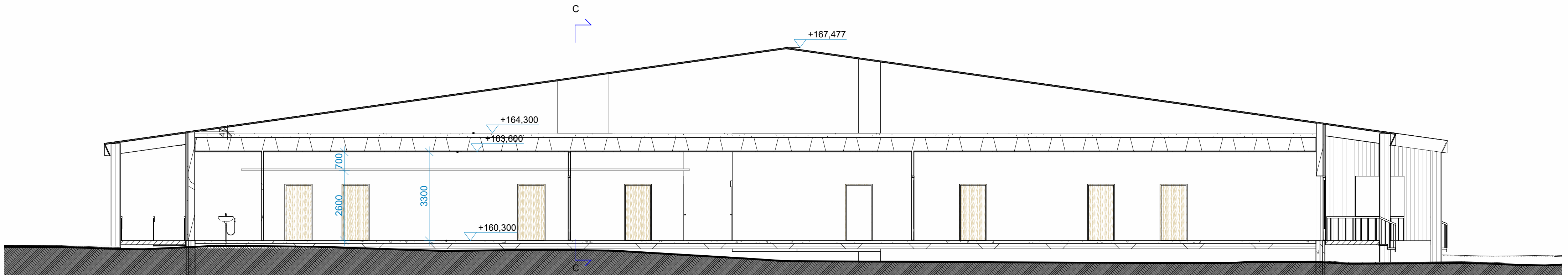
Leikkaus A-A 1 : 100
