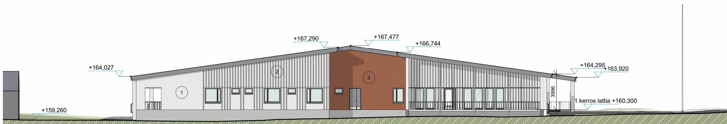
Julkisivu koilliseen 1 : 200
